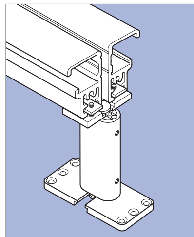
Podpěrná konzole vodička
